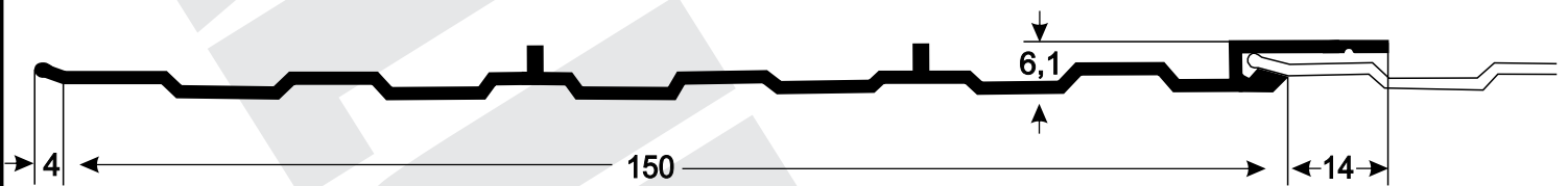
Y-354 0,866 kg/m
