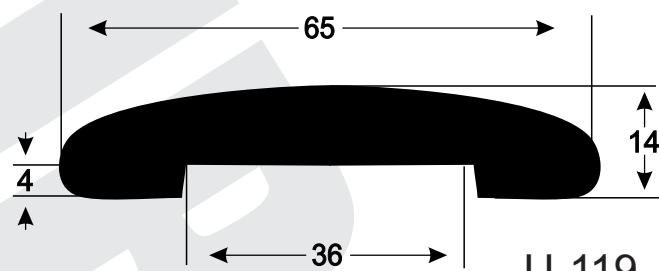
U-119 1,693 kg/m
