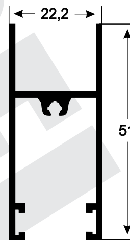
SU-187 0,534 kg/m
