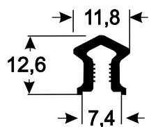
U-873 0,133 kg/m
