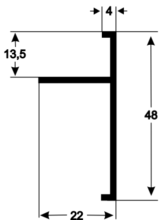
T-105 0,300 kg/m
