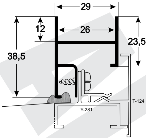
Y-283 0,470 kg/m
