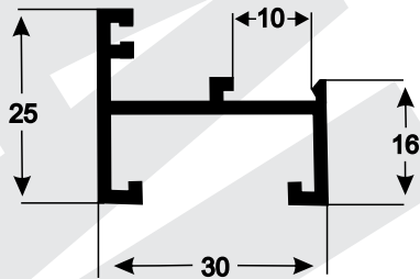
Y-113 0,345 kg/m
