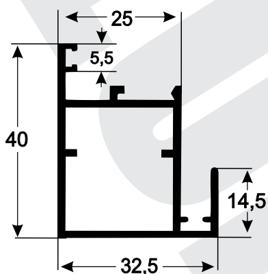
P-151 0,610 kg/m
