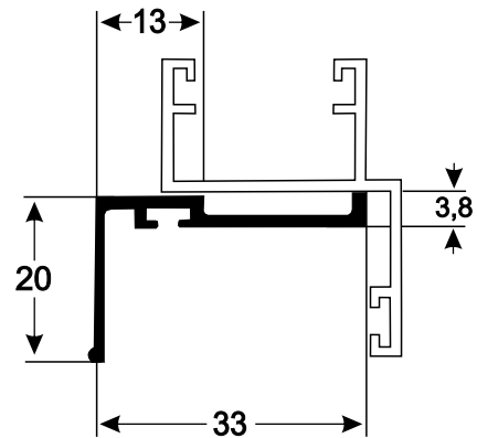
L-387 0,220 kg/m
