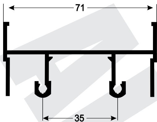
SU-001 0,773 kg/m
