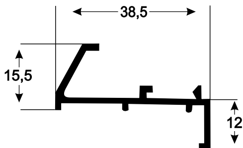
Z-063 0,325 kg/m
