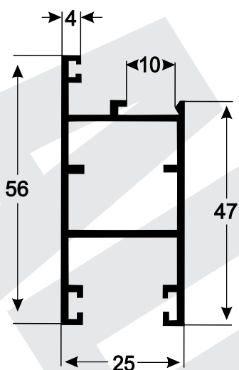
A-048 0,710 kg/m
