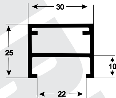
A-057 0,470 kg/m
