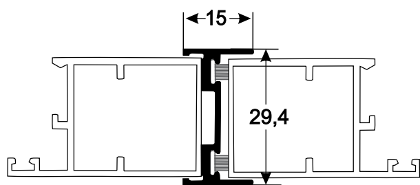
I-105 0,263 kg/m
