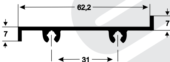
Z-195 0,412 kg/m
