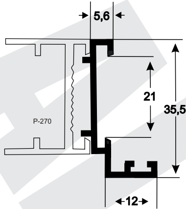
L-519 0,300 kg/m
