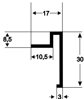
L-469 0,179 kg/m
