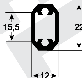
D-070 0,263 kg/m
