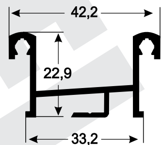
SU-272 0,430 kg/m
