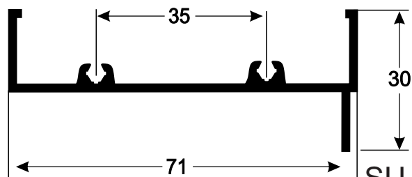
SU-004 0,526 kg/m
