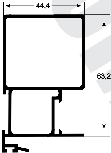
SU-049 0,997 kg/m
