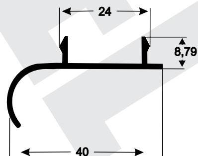
L-570 0,288 kg/m
