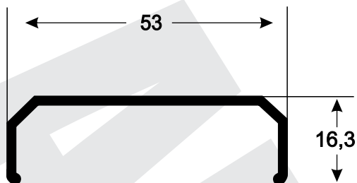
U-498 0,285 kg/m
