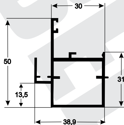
P-277 0,724 kg/m
