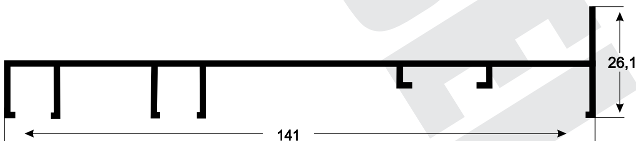
SU-123 0,917 kg/m
