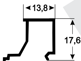
SU-103 0,156 kg/m
