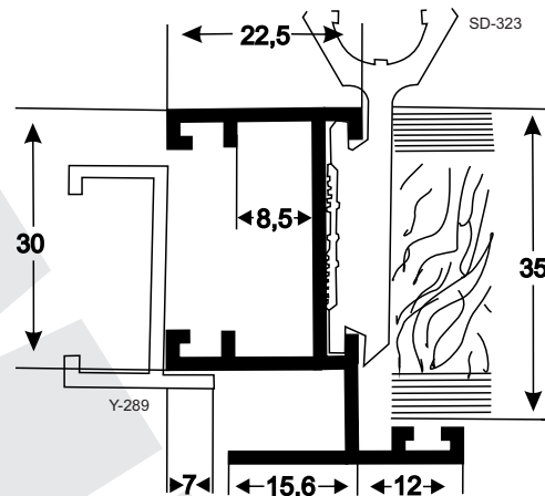
Y-342 0,575 kg/m
