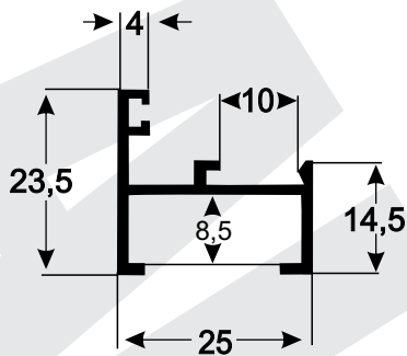
Y-197 0,298 kg/m
