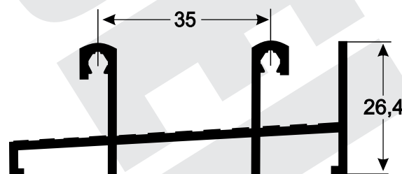
E-578 0,707 kg/m
