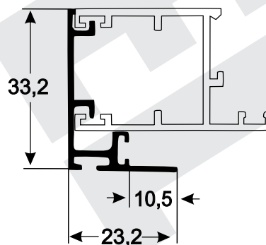
L-498 0,318 kg/m
