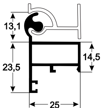
P-161 0,495 kg/m
