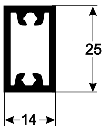
D-082 0,356 kg/m
