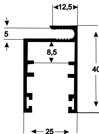
Y-312 0,550 kg/m
