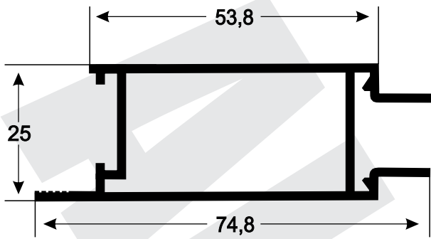
SU-224 0,685 kg/m
