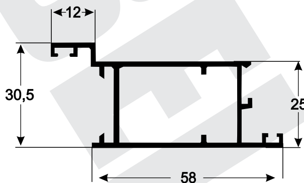
P-415 0,797 kg/m
