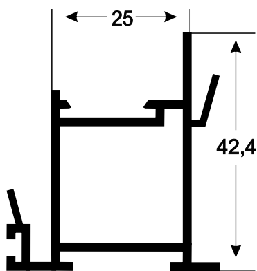
SU-042 0,589 kg/m
