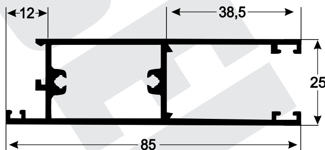
A-139 1,033 kg/m
