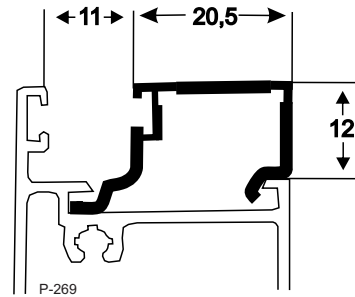
U-679 0,180 kg/m
