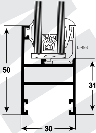
A-088 0,650 kg/m
