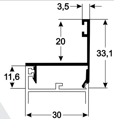
Y-201 0,290 kg/m
