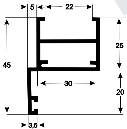
P-156 0,600 kg/m
