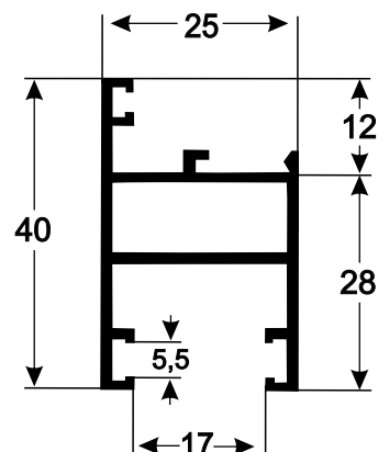
A-047 0,560 kg/m
