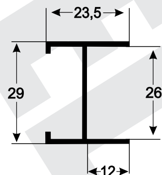
I-090 0,300 kg/m
