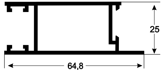
SU-245 0,634 kg/m
