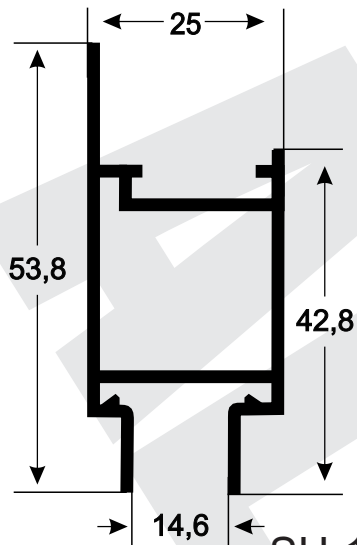
SU-192 0,554 kg/m
