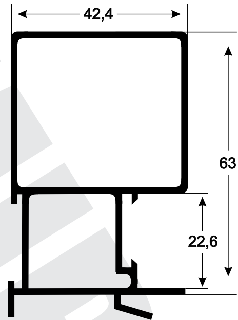
SU-047 1,041 kg/m
