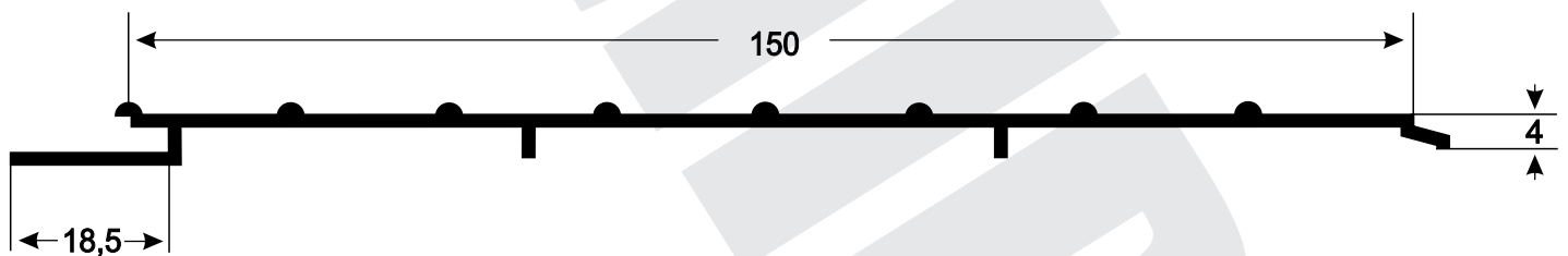
Y-430 0,686 kg/m
