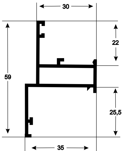
P-406 0,612 kg/m
